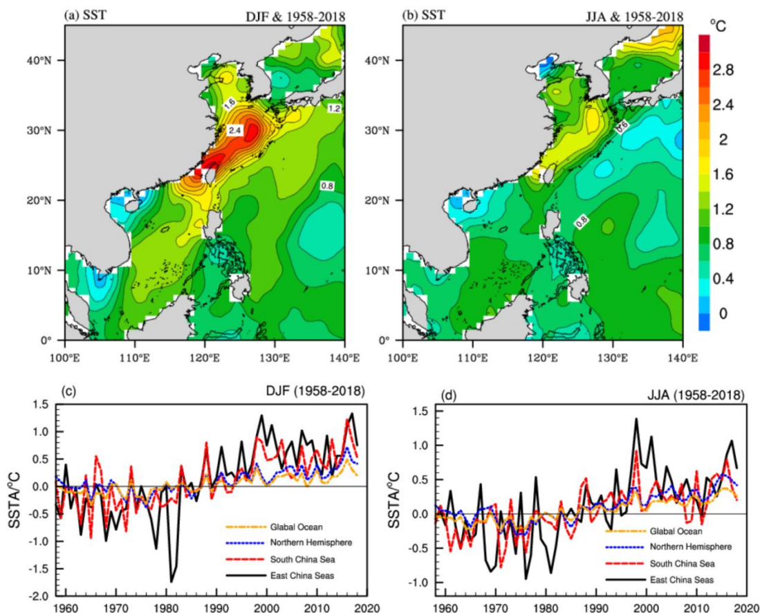
图 3-13 1958—2018 年冬、夏季渤海、黄海、东海和南海的 SST 线性上升幅度 (a、b, 单位: °C) 及距平时间序列 (c、d, 单位: °C) [30]
