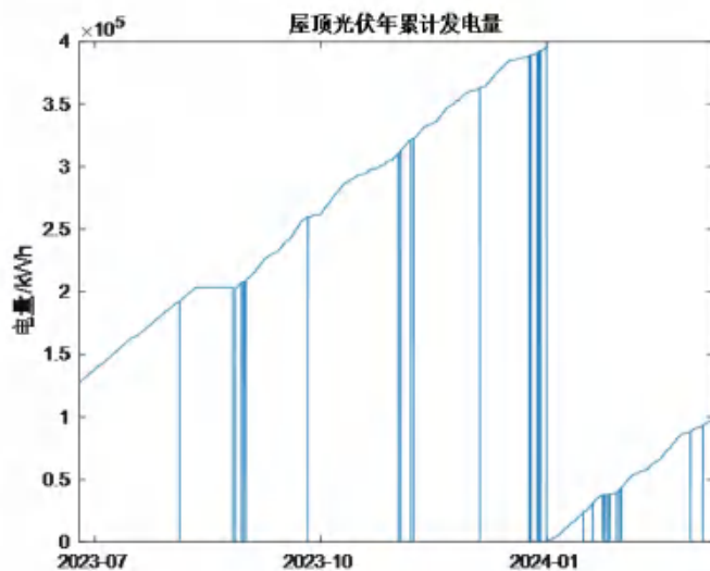
图6 新闻中心光储直柔光伏发电量
