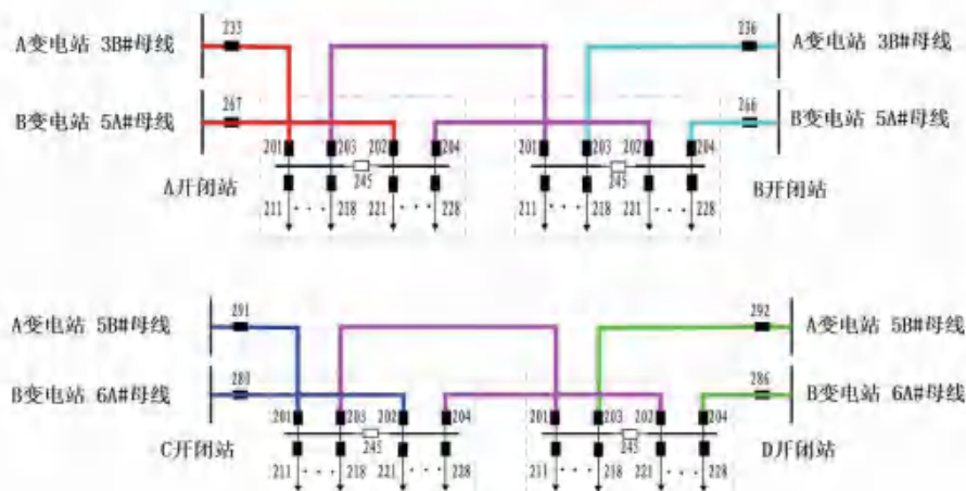
图6 城市绿心双环网合环运行网架结构示意图
