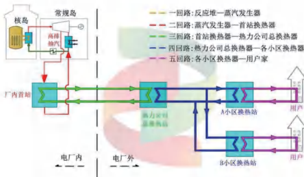
图 4 核能供暖工程系统原理图
