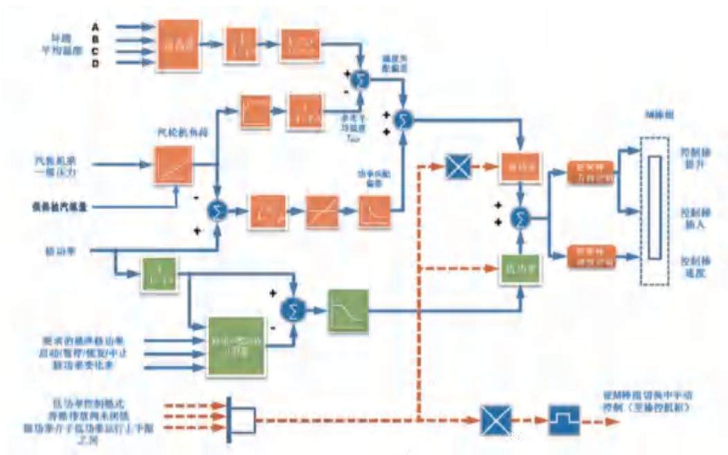
图7 堆-机-电-热协调控制逻辑图
