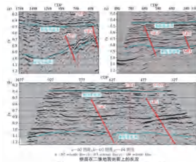
图4 断层在二位地震剖面上的反应
