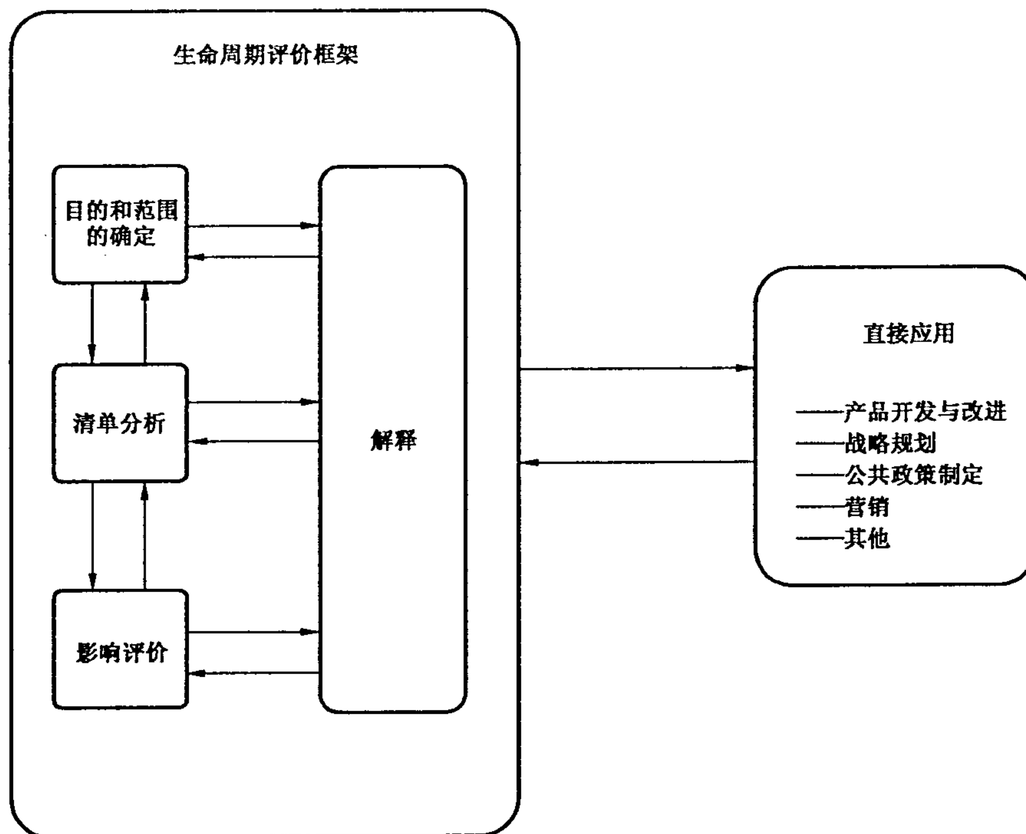
图 1 LCA 的阶段
